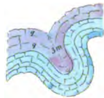
Fig. 6. Quarzitbiegung am Gstellhorn.
